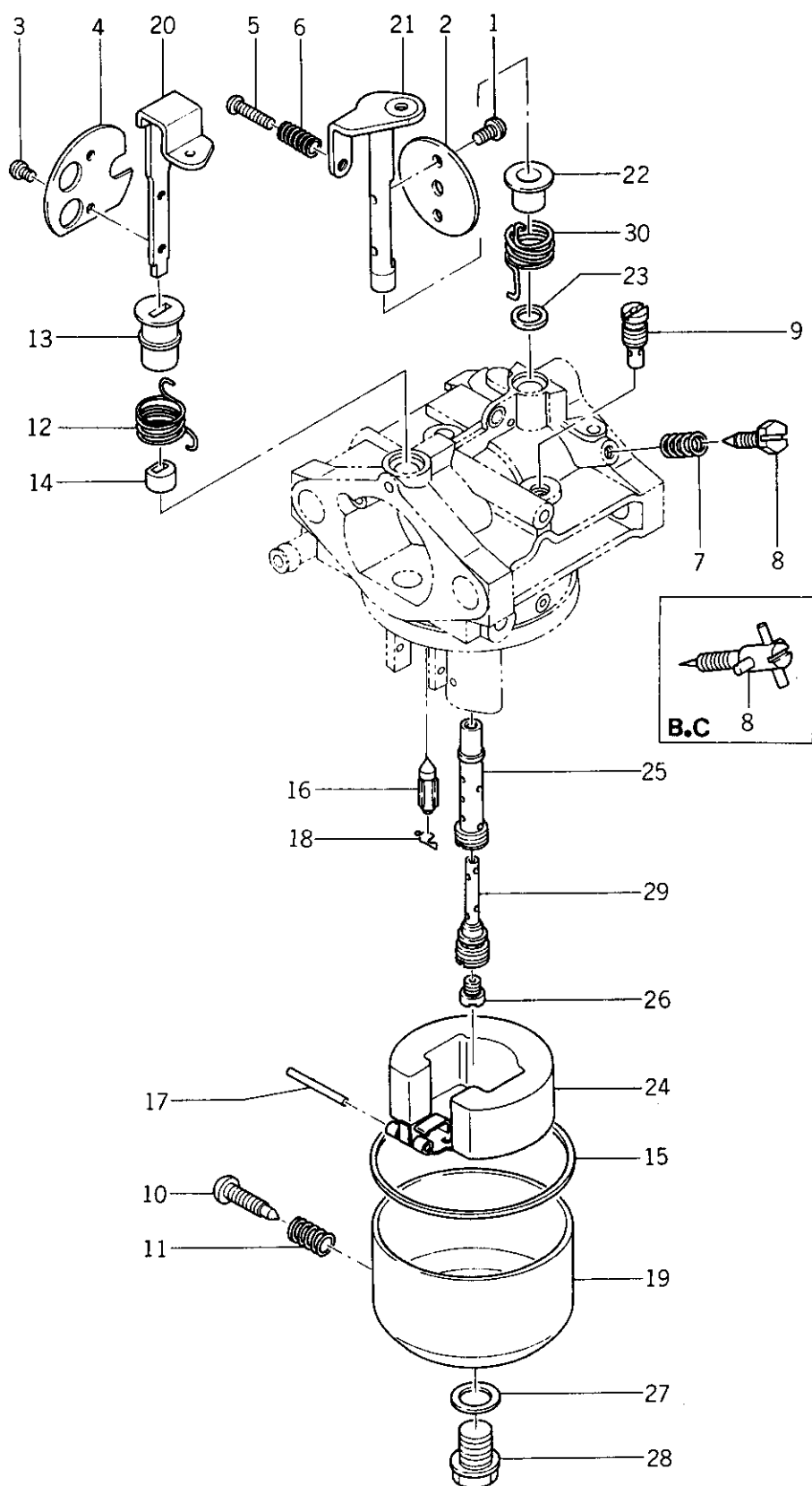
Fig. C-1 CARBURETOR
